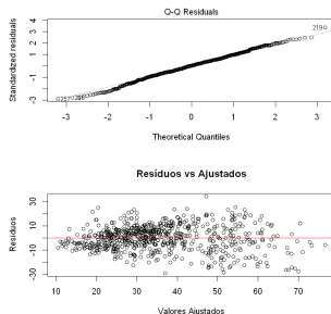
Figura 3: QQ-plot e resíduos vs valores ajustados
